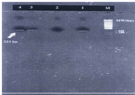
شکل ۱- نتایج PCR در مورد نمونه‌های بالینی شماره ۳ و ۴، نمونه‌های بالینی که نتیجه PCR آنها مثبت گزارش شد. شماره ۲، کنترل منفی. شماره ۱، کنترل مثبت.
